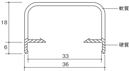
KTパッキング
