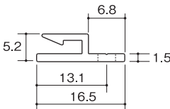
KT用アルミレール
